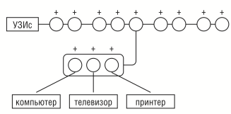
Рис. 8. Расширение зоны обслуживания удлинителем (пример).
