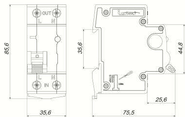
Рис. 3. Размеры УЗДП
